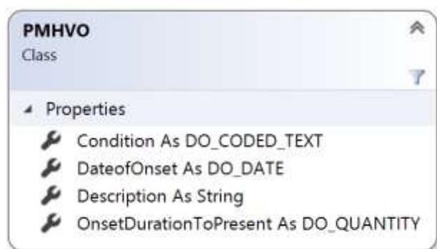
شکل ۲۳ - کلاس PMHVO
