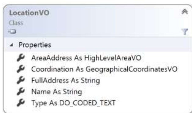
شکل ۱۱- کلاس LocationVO
