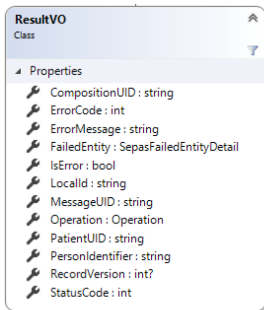
شکل ۳۶ - کلاس ResultVO
