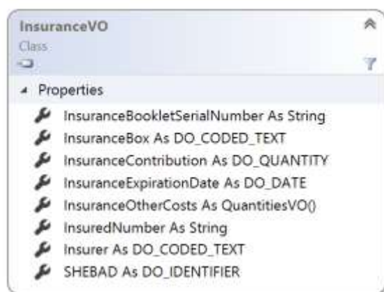
شکل ۱۵- کلاس insuranceVO
