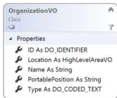
شکل ۴- کلاس OrganizationVO
