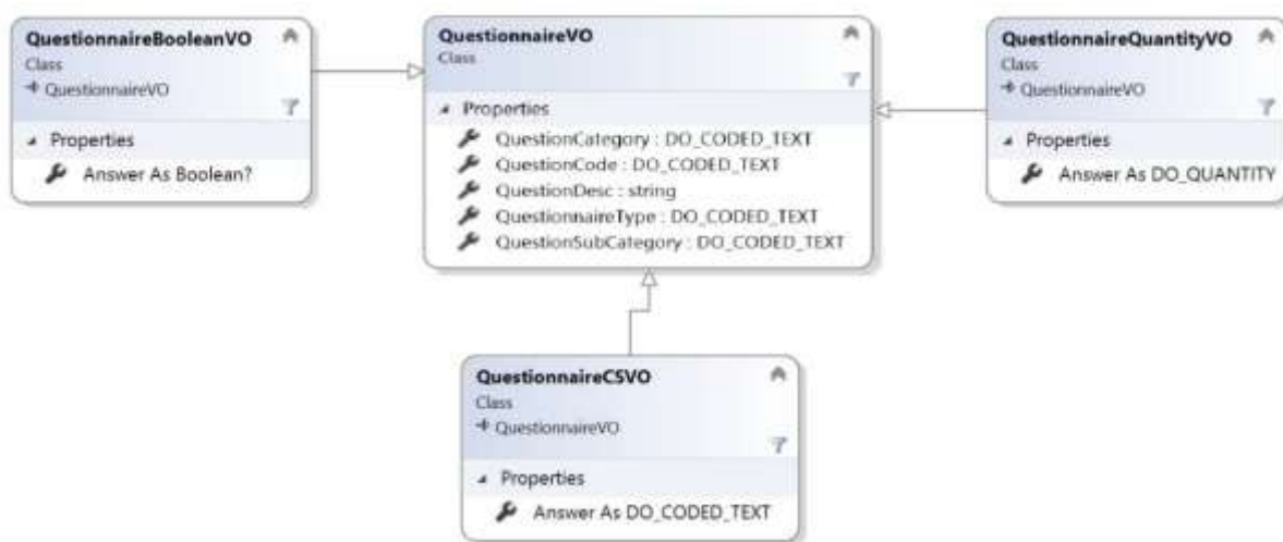
شکل ۲۸ - کلاس QuestionnaireVO
