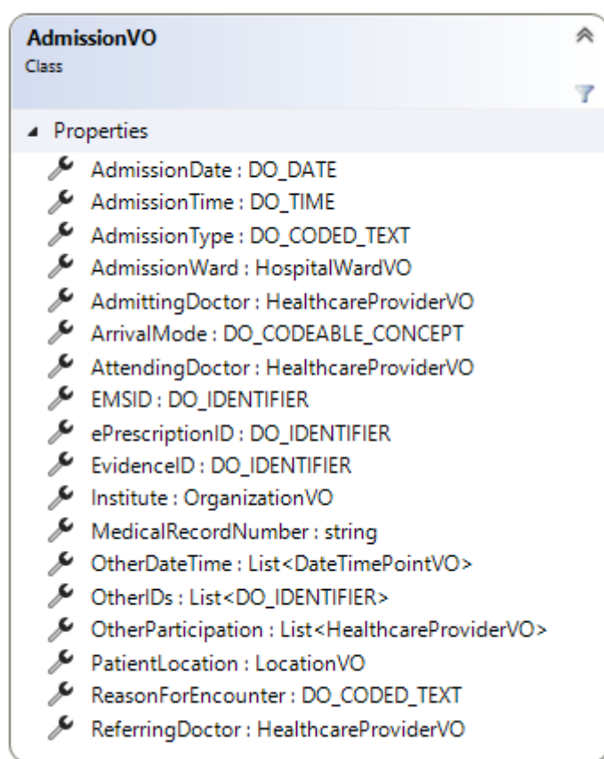
شکل ۳ - کلاس AdmissionVO
