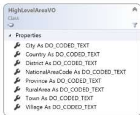
شکل ۵ - کلاس HighLevelAreaVO
