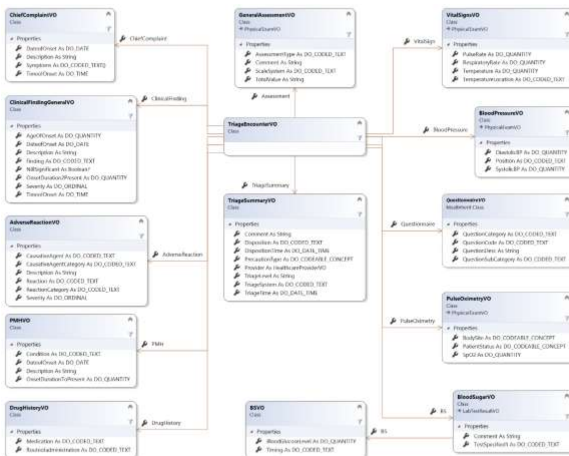
شکل ۲۱- جزئیات TriageEncounterVO
