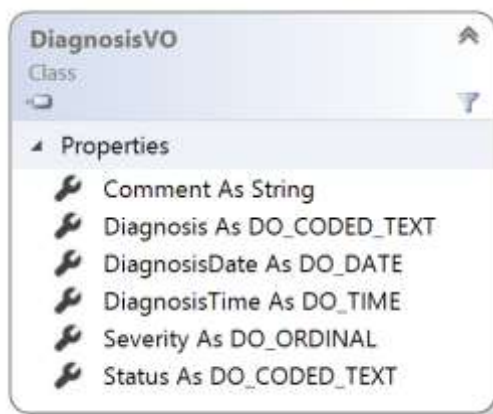
شکل ۱۶- کلاس DiagnosisVO
