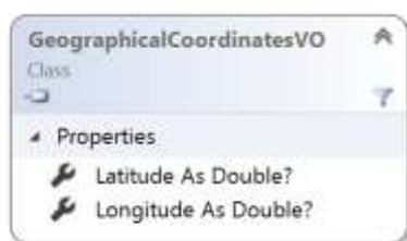
شکل ۱۲ - کلاس GeographicalCoordinatesVO
