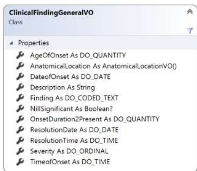
شکل ۲۵ - کلاس ClinicalFindingGeneralVO
