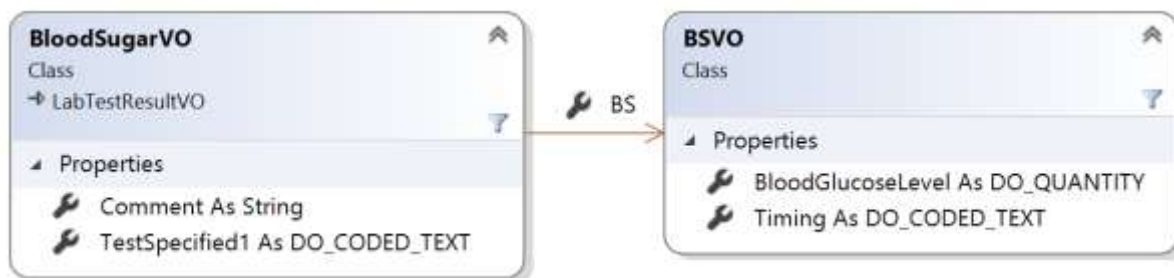
شکل ۳۰ - کلاس BloodSugarVO
