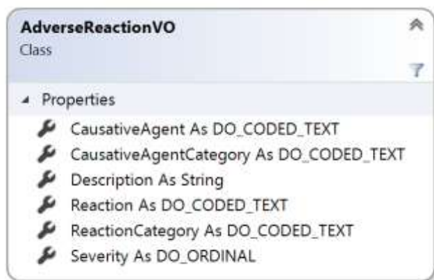
شکل ۲۷- کلاس AdverseReactionVO
